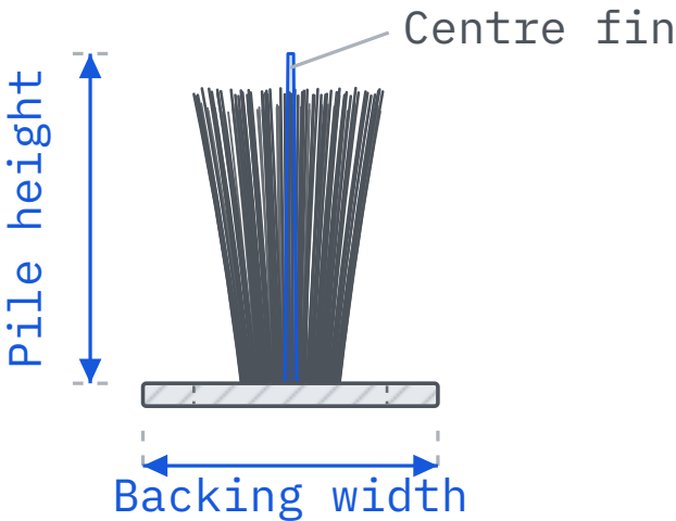
Fin seal · filament plus centre film
